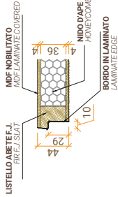
DETTAGLIO SEZIONE PANNELLO LEAF DETAIL SECTION
