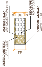
DETTAGLIO SEZIONE PANNELLO LEAF DETAIL SECTION
